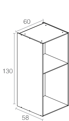
Módulo Semicolumna
